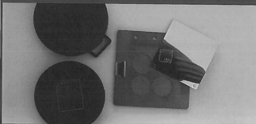
Figuur 9 Gedemonteerde radon- (links) en thorondochterdetector (rechts).
