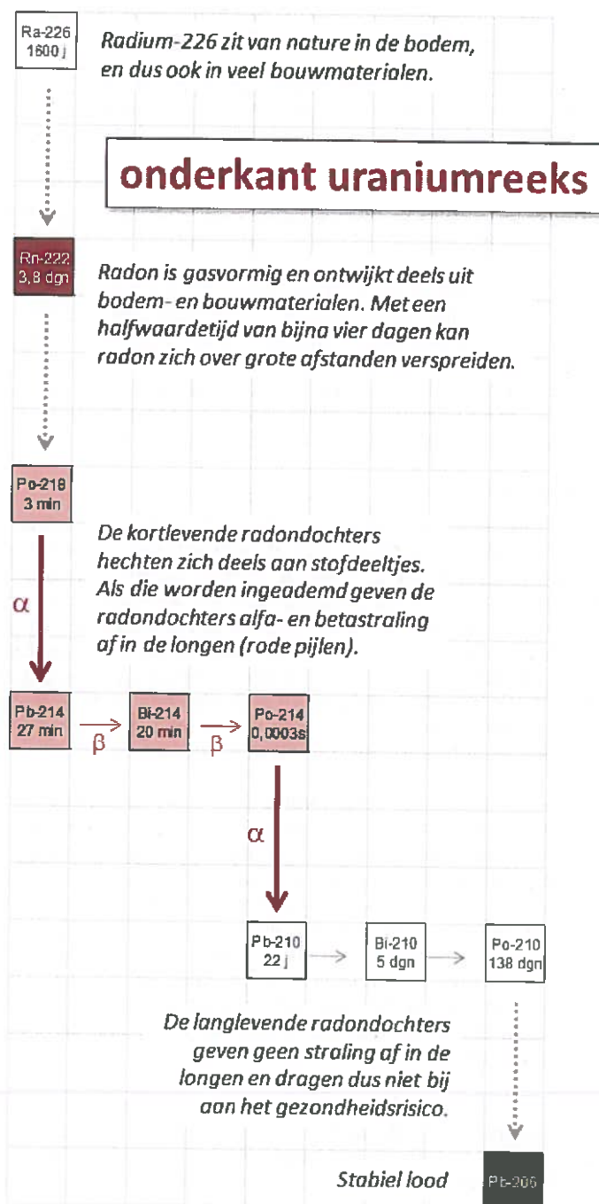
Figuur 3 Onderste gedeelte van de natuurlijke vervalreeks van uranium.
