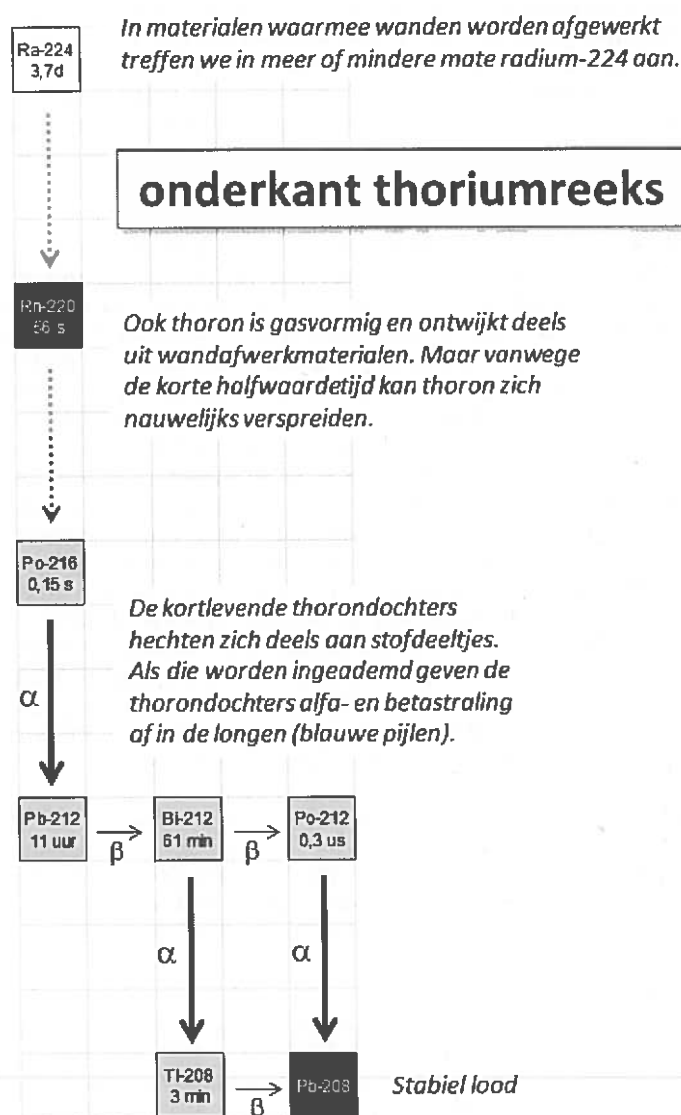
Figuur 4 Onderste gedeelte van de natuurlijke vervalreeks van thorium.
