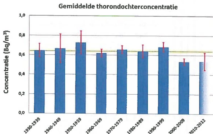
Figuur 15 Gemiddelde thorondochterconcentratie per bouwperiode.
