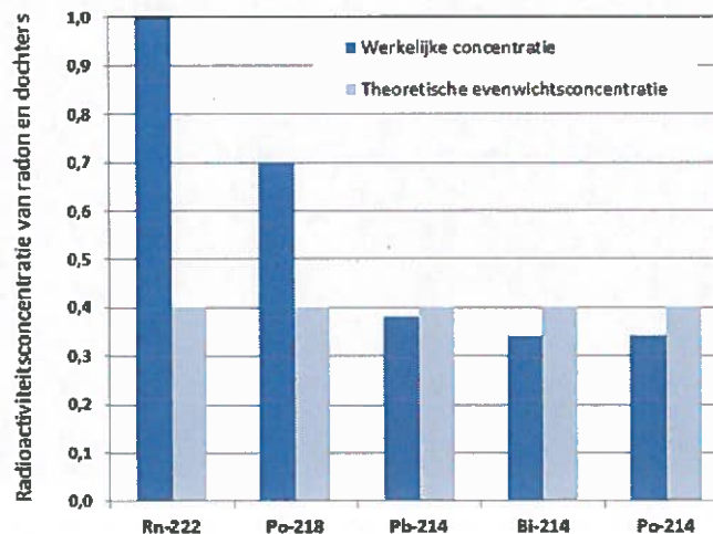
Figuur 7 Voorbeeld van de radioactiviteitsconcentratie in lucht van de kortlevende radonochters, ten opzichte van radon zelf.
